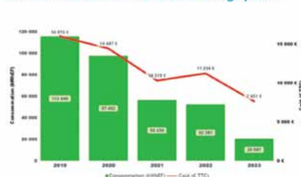
Evolution des consommations d'éclairage public
